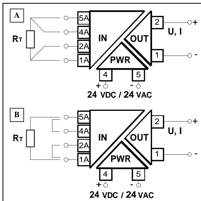
Rys. 2) Sposób podłączenia czujnika do przetwornika:
